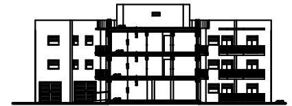
Sezione B-B'
